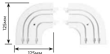
Поворот трехрядный «Стандарт»
