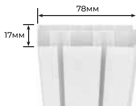
ГАБАРИТЫ ШИНЫ
